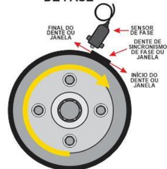
RODA COM 1 DENTE OU 1 JANELA
