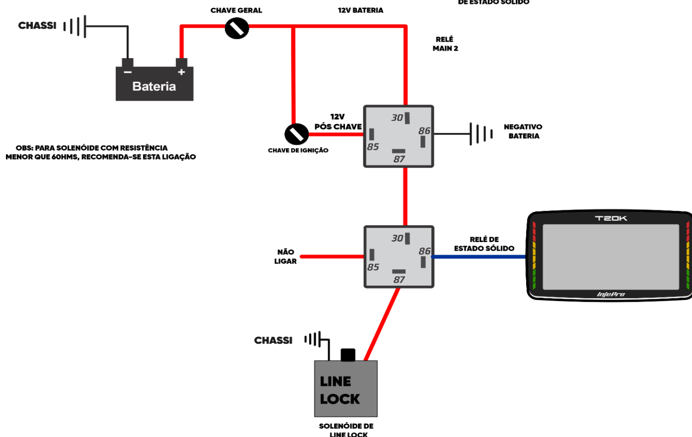
ESQUEMA DE LIGAÇÃO PARA LINE-LOCK B&M COM RELÉ DE ESTADO SÓLIDO
